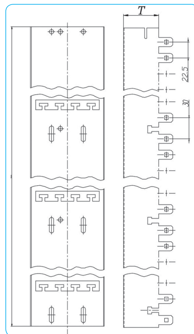
Монтажный хомут «LSA-PLUS 2/10» без перфорации
